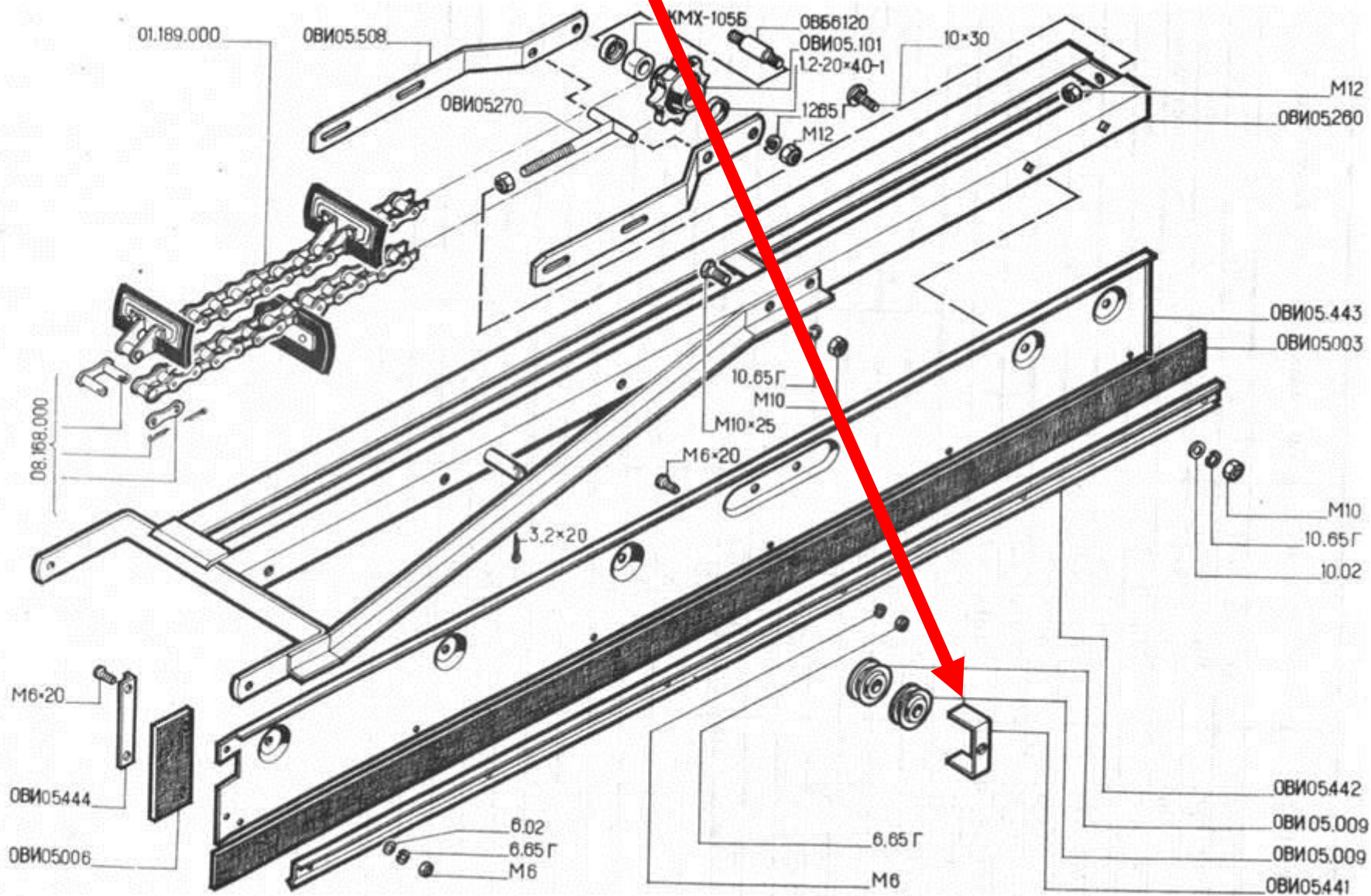
Рис. 26. Питатель ОВИ 05.200.
